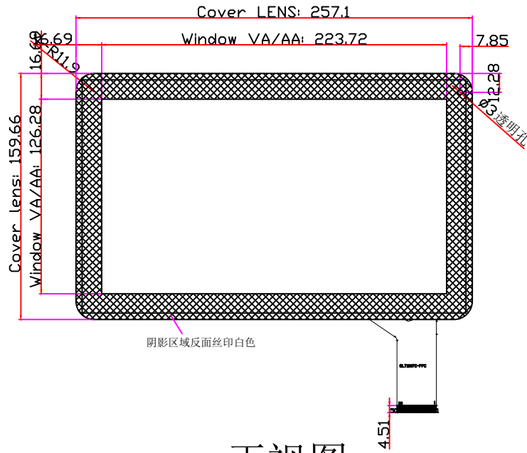
正视图
