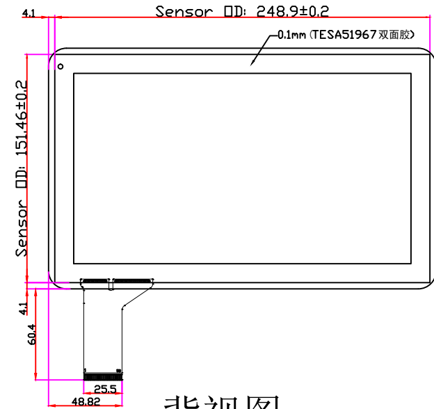
背视图
