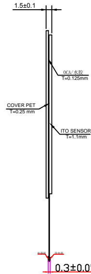
侧视图
